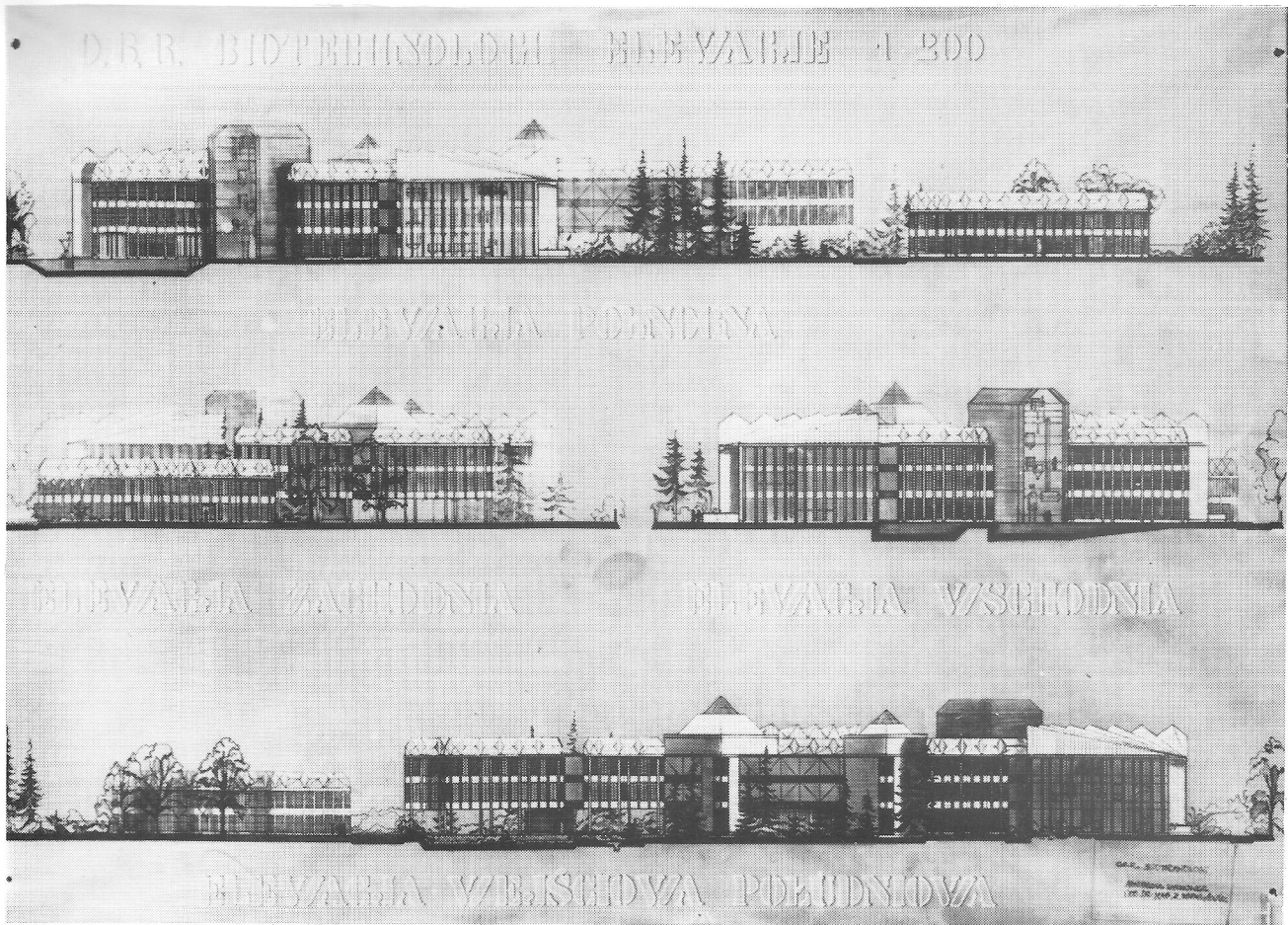
Ośrodek badawczo-rozwojowy biotechniki arch. Agnieszka Sychowicz-Bulska, Politechnika Warszawska
