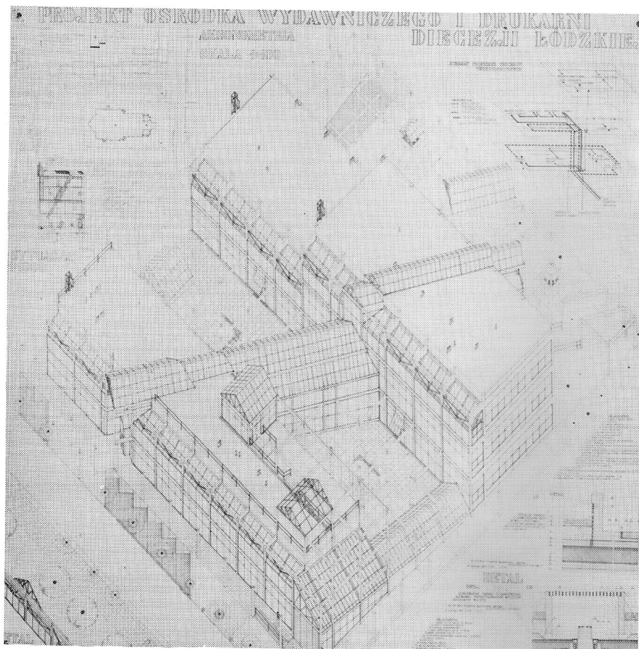
Projekt Ośrodka Wydawniczego i Drukarni Diecezjalnej arch. Roman Staszewski, Politechnika Łódzka
