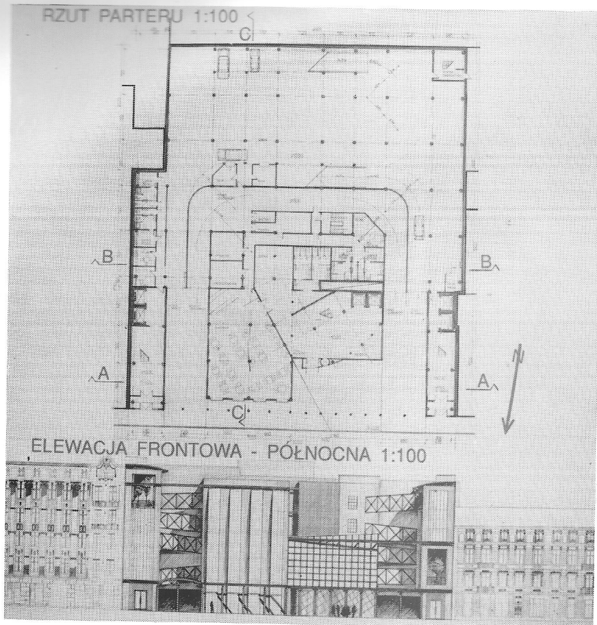
Wielopoziomowy garaż w centrum Łodzi. arch. Anna Diehl, Politechnika Łódzka
