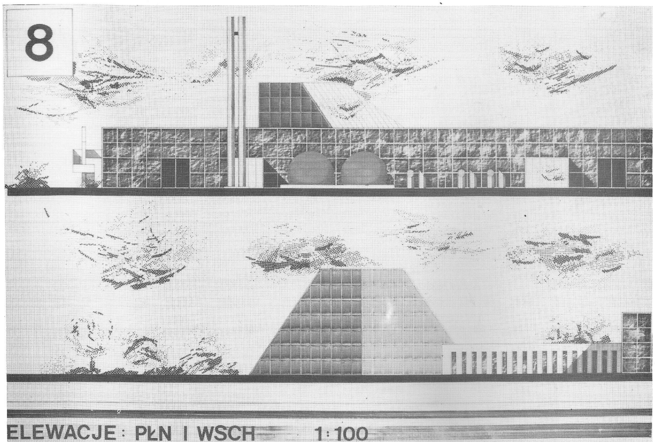
Fabryka artykułów gospodarstwa domowego arch. Tomasz Kazimierzczak, Politechnika Szczecińska
